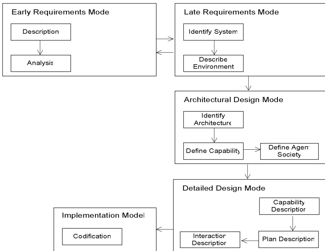
Figura 1: La metodologia Tropos
