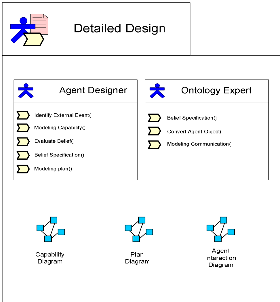
Figura 21. Descrizione della fase Detailed Design rappresentata come una disciplina SPEM
